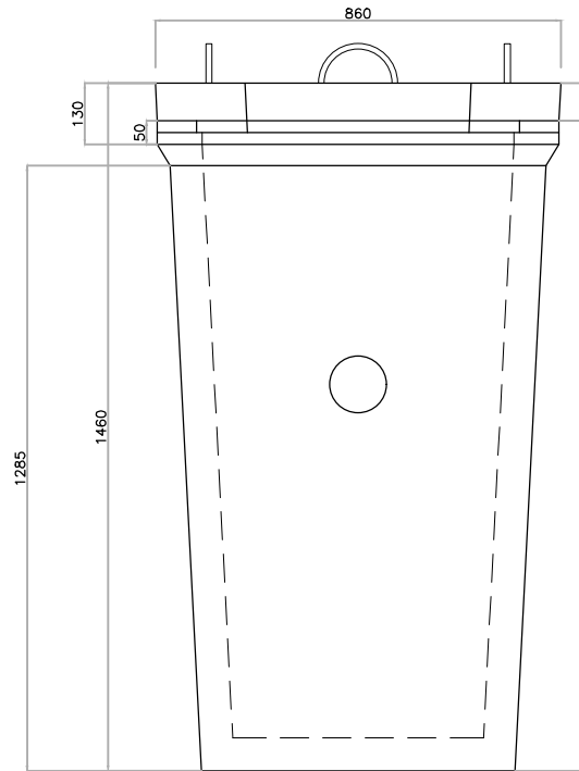
ELEVATION
